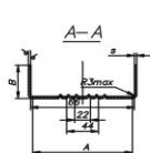
Термопрофиль гнутый П-образный / ТПП
