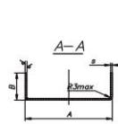
Профиль гнутый П-образный / ПП
